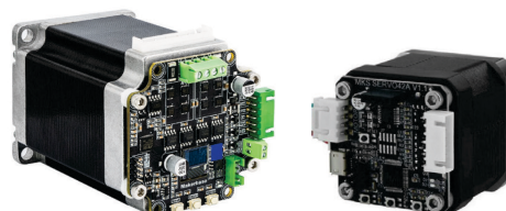
а) драйвер за NEMA23 б) драйвер за NEMA17
