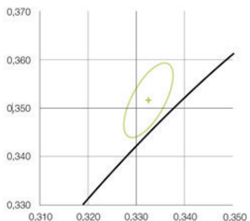
Фиг. 8. Относителни цветови координати на LED със студено-бяла светлина (5700K)
