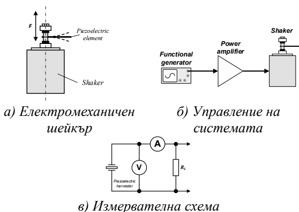
Фиг. 4. Базов експериментална установка
