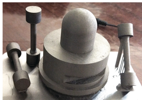
Фиг. 6. Детайл „Сърце-дюза“, изработен на 3D принтер за метал ProX DMP200
