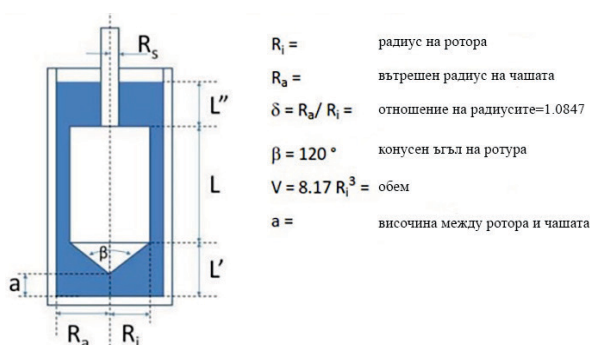
Фиг. 3. Геометрия на ротора и чашата.
