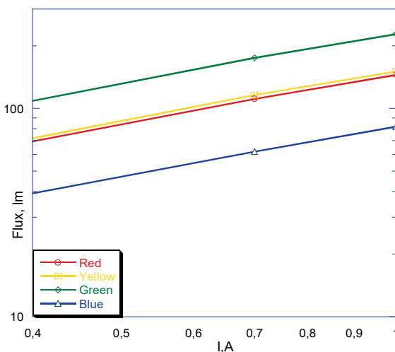
Фиг. 5. Изменение на светлинния поток на LED в зависимост от протичащия ток
