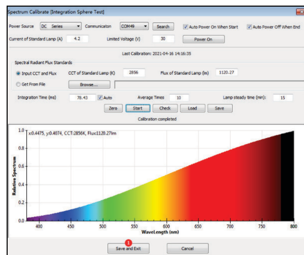
Фиг. 10. Спектрално разпределение на еталонна лампа
