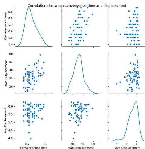
Фиг. 8. Шестнадесет WMRs: корелация между времето на конвергенция и средното и максимално изместване
