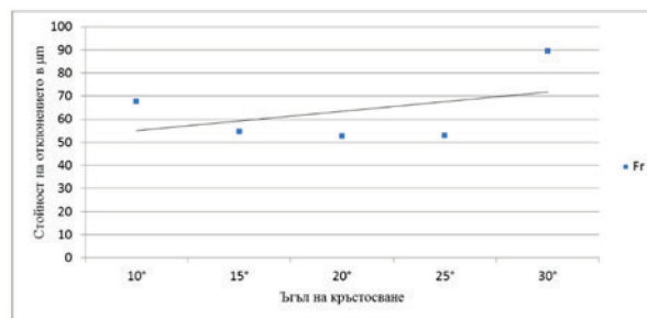
Фиг. 6. Грешка от радиално биене
