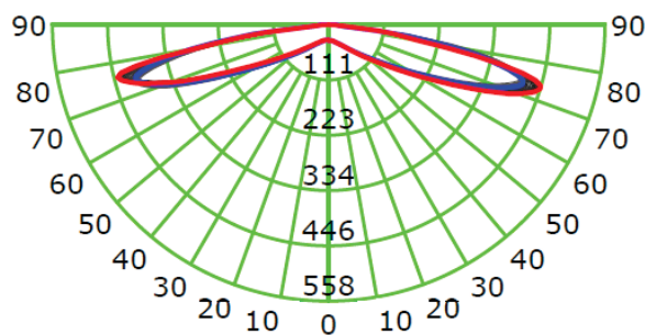
Фиг. 9. Измерени светлоразпределения на LED осветител 12 W за рекламно осветление
