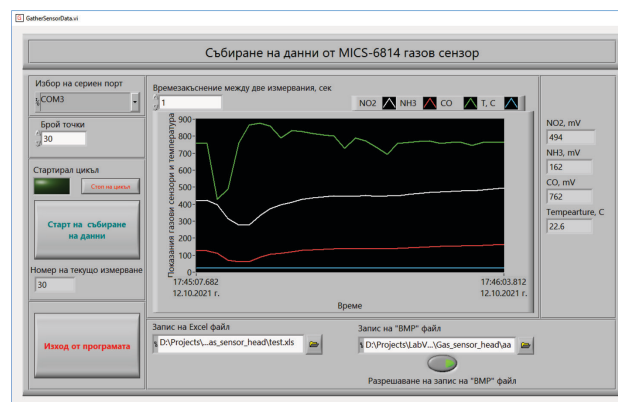
Фиг. 3. Програма за събиране на данни
