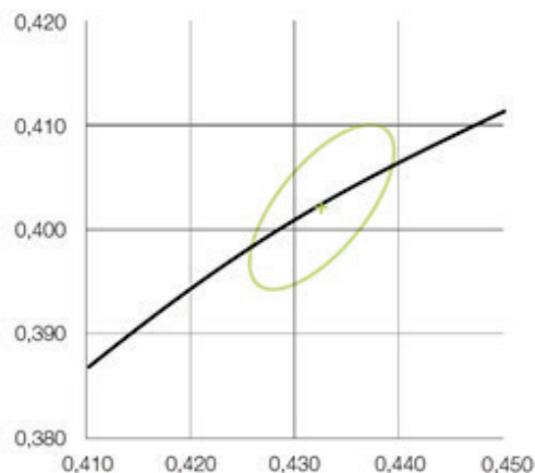
Фиг. 6. Относителни цветови координати на LED с топло-бяла светлина (3000K)
