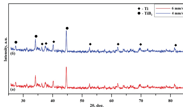
Фиг. 3. Рентгенова дифрактограма на получените образци.
