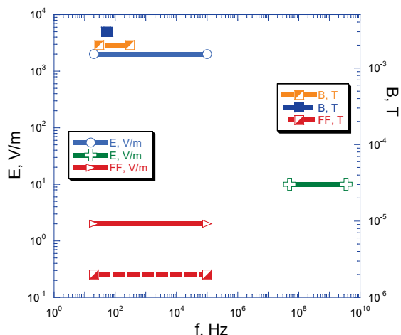
Фиг. 2. Честотен диапазон на уредите за измерване на ЕМИ
