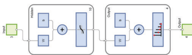
Фиг. 7. Структура на невронната мрежа за класификация
