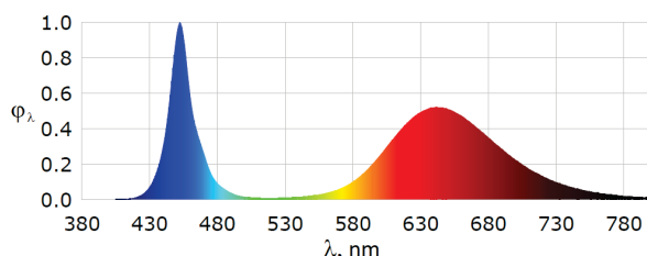
Фиг. 14. Спектрално разпределение на LED осветител 12 W оранжерийно осветление
