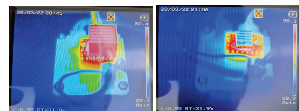
Фиг. 4. Топлинен режим на драйверите в номинален работен режим
