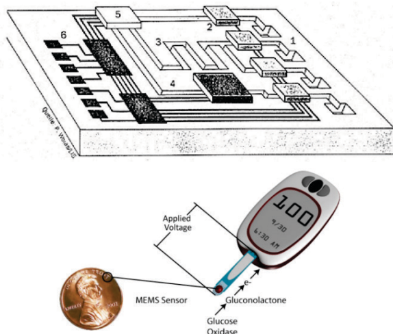
Фиг. 5. Микросистема, изработена с прилагане на йонно-лъчево ецване. Био- MEMC на Southwest Center for Microsystems Education (образование)
