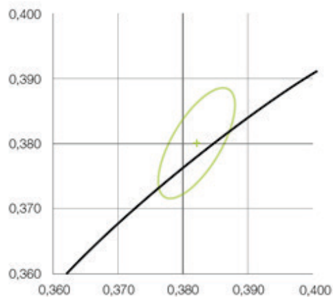
Фиг. 7. Относителни цветови координати на LED с бяла светлина (4000K)
