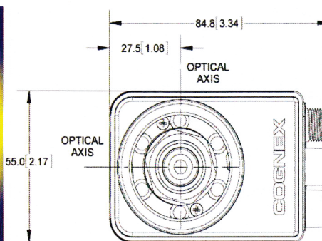
Фигура 7 камера COGNEX In-Sight 7402C и физическите ѝ размери.
