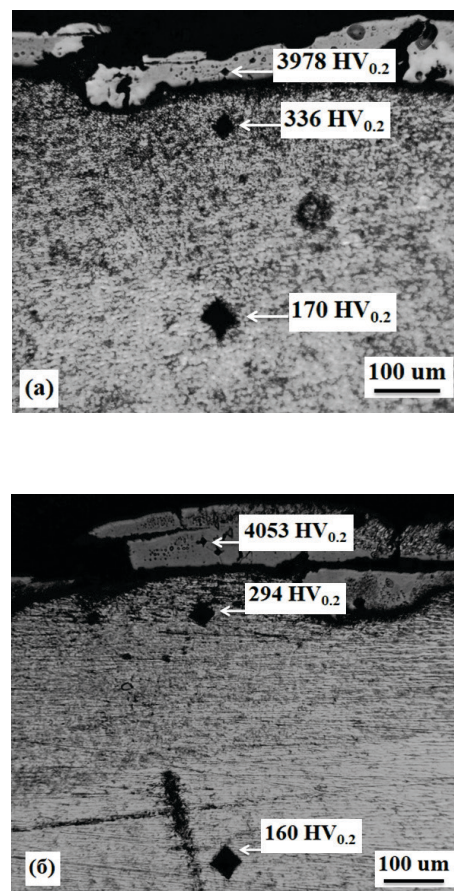
Фиг. 4. Измерване на микротвърдост на образците със скорост на движение на образца : а) 6 mm/s ; б) 4 mm/s
