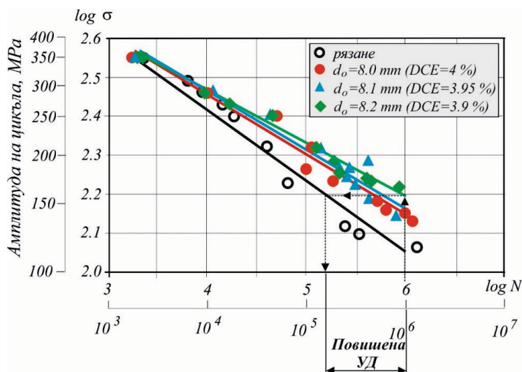
Фиг. 4. S-N криви
