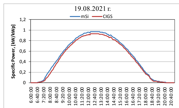
Фиг. 8. Изменение на специфичната мощност за PV подсистеми от mSi и CIGS за 19.08.2021 г.
