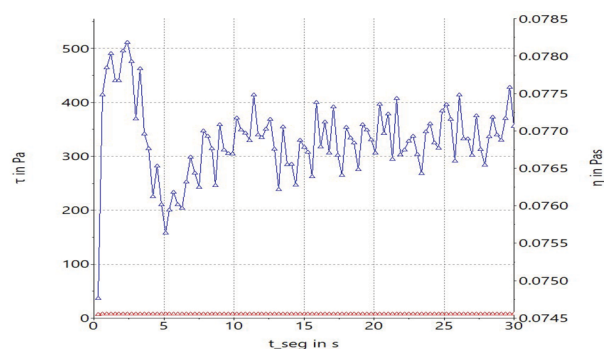
Фиг. 6. Реограма на вискозност при 20 °C.
