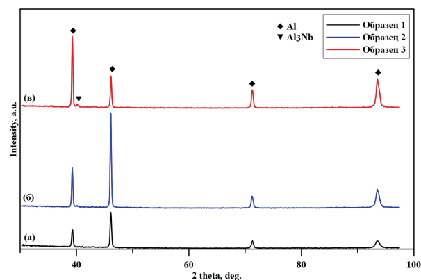
Фиг. 2. Рентгеноструктурен анализ на електронно-лъчево заварените образци
