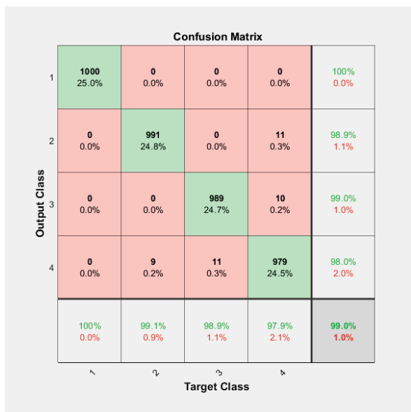
Фиг. 9. Матрица на резултатите на обучени ANN с възможности за класификация
