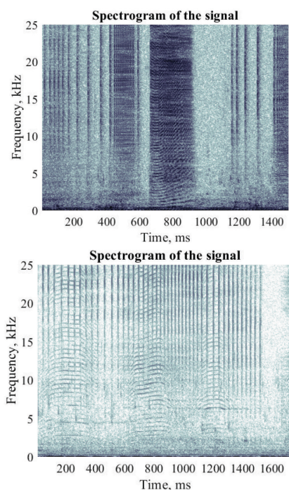
Фиг. 5. Спектрограми на анализирани сигнали от делфини. Горе – на бърст сигнал, долу – на клик сигнал.
