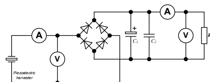
Фиг. 5. Експериментална установка с изправител
