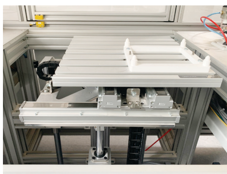
Фиг. 7. Серво-маса
