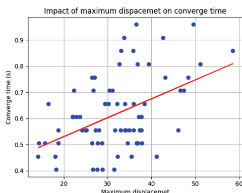
Фиг. 9. Шестнадесет WMR: Влияние на максималното изместване върху времето за конвергенция
